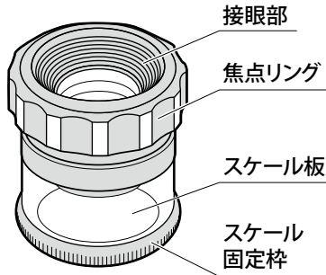
■NSL-15-1 スケール板
