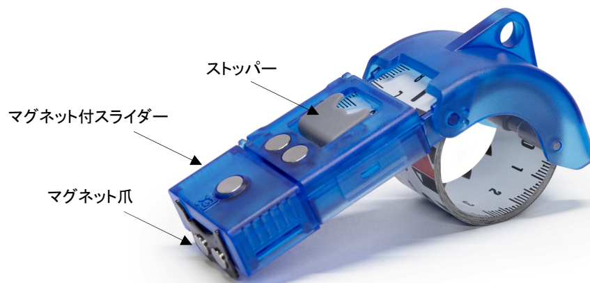
写真1 くるくるメジャーPro（商品名：スパイラルメジャー クイック）
